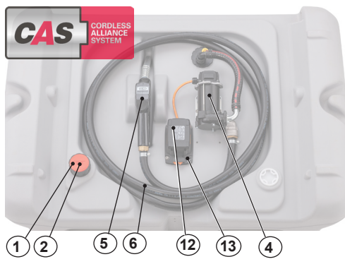
Widok wnętrza DT-Mobil Easy 440 I
