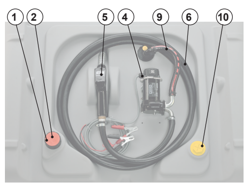
DT-Mobil Easy 440 I con pompa 12V 40 l/min
